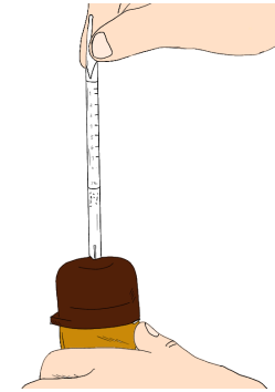
検知管を回してキズをつけ、折る。
